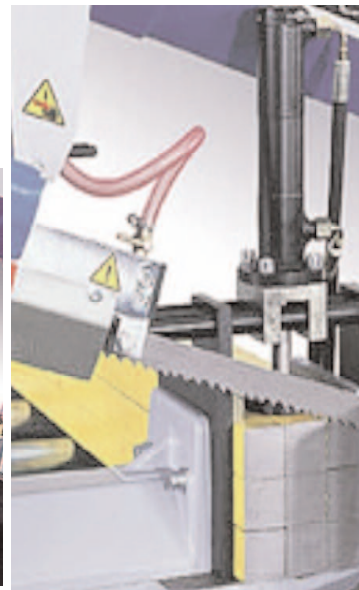
Vertikalspannsystem hydraulisch
