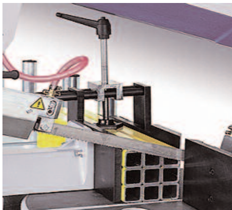
Vertikalspannsystem manuell
