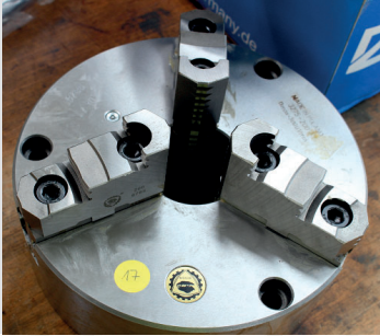
Nr. 17: Dreibacken-Drehfutter BISON; Ø 200 mm; Guss; DIN 6350
