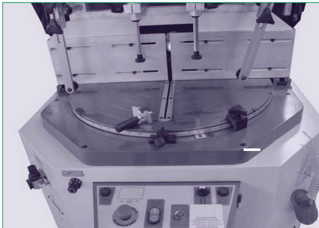
Materialspanner 4-fach einzeln verschiebbar und wegklappbar
